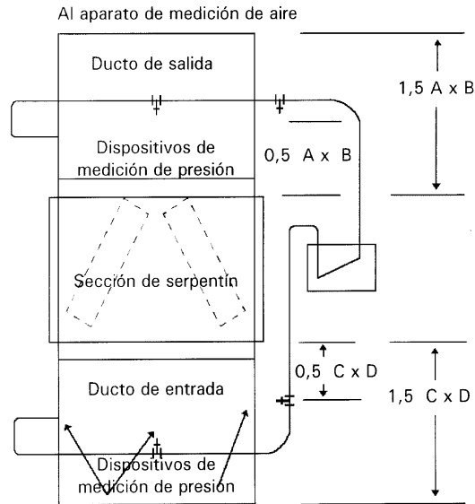
Figura 7. Medición de la presión estática externa
